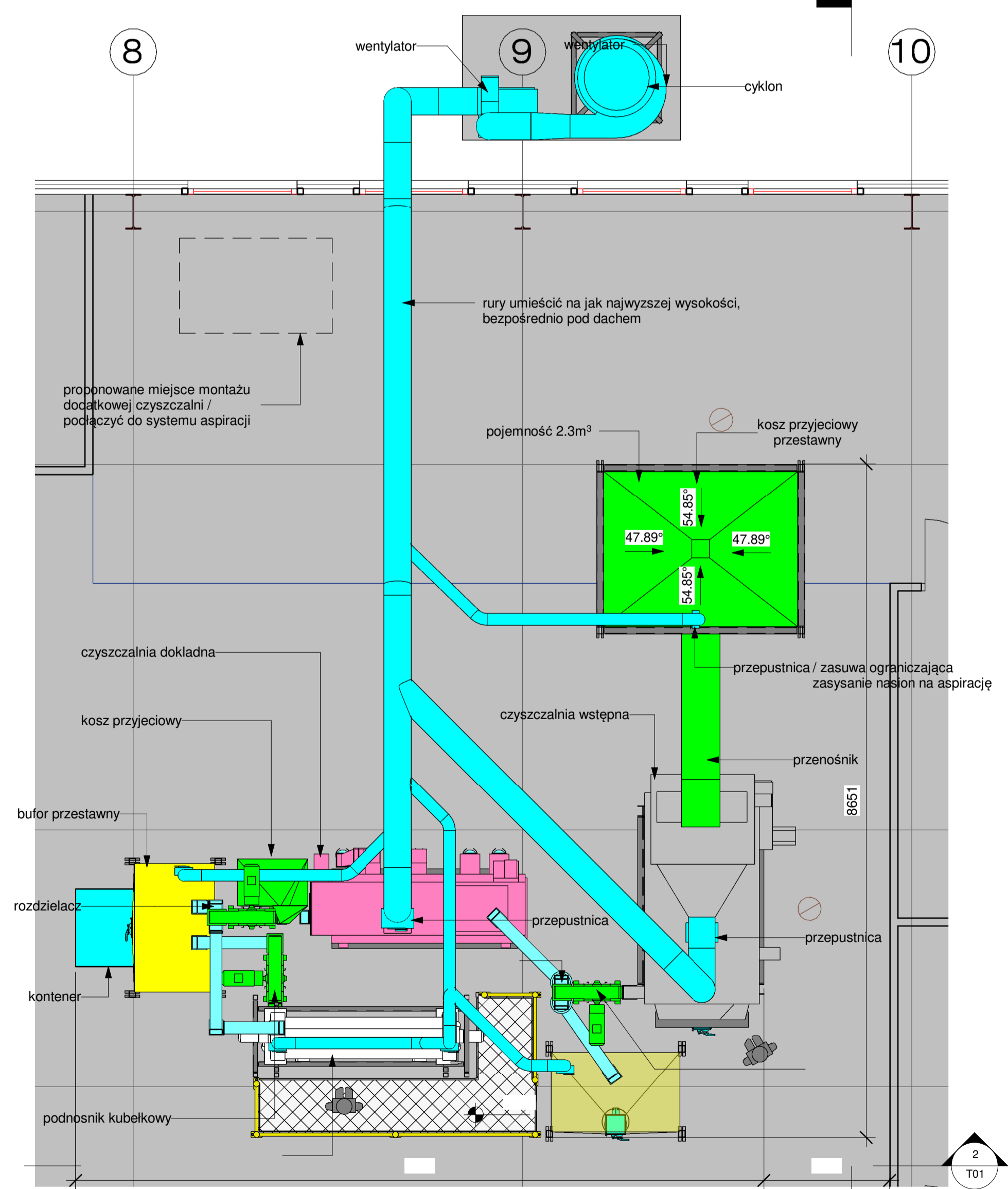
1 Poziom 2 1 : 50
