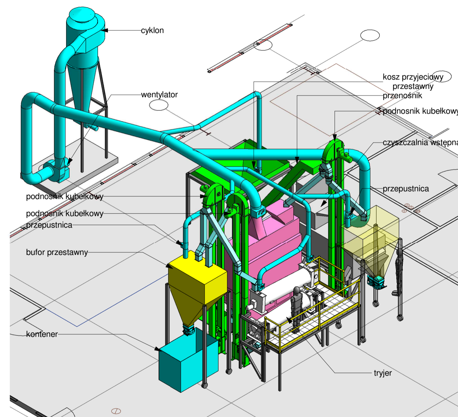
4 Aksonometria_2
