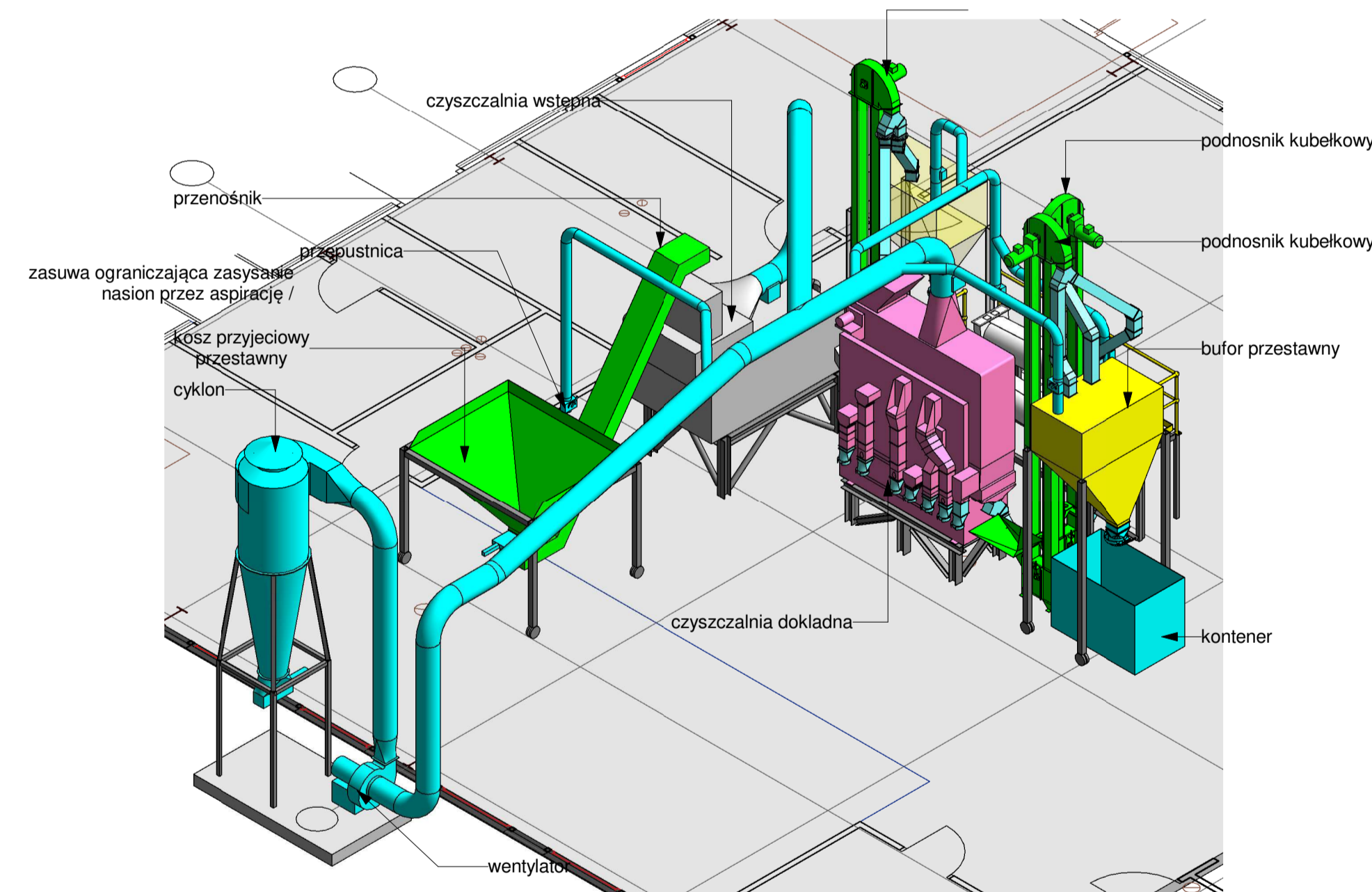
3 Aksonometria_1
