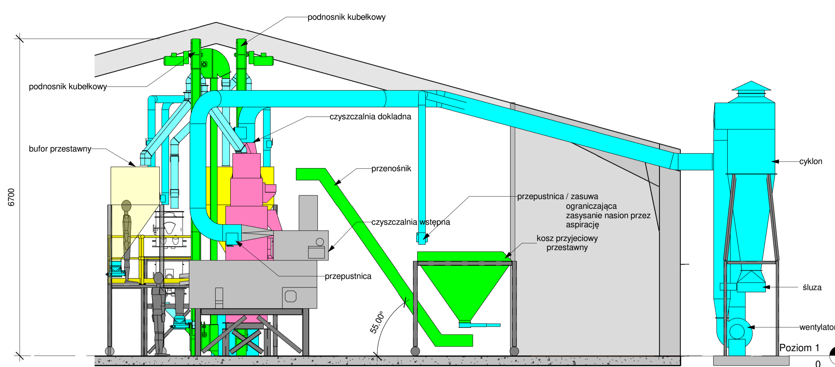
5 Przekrój 1 1 : 50
