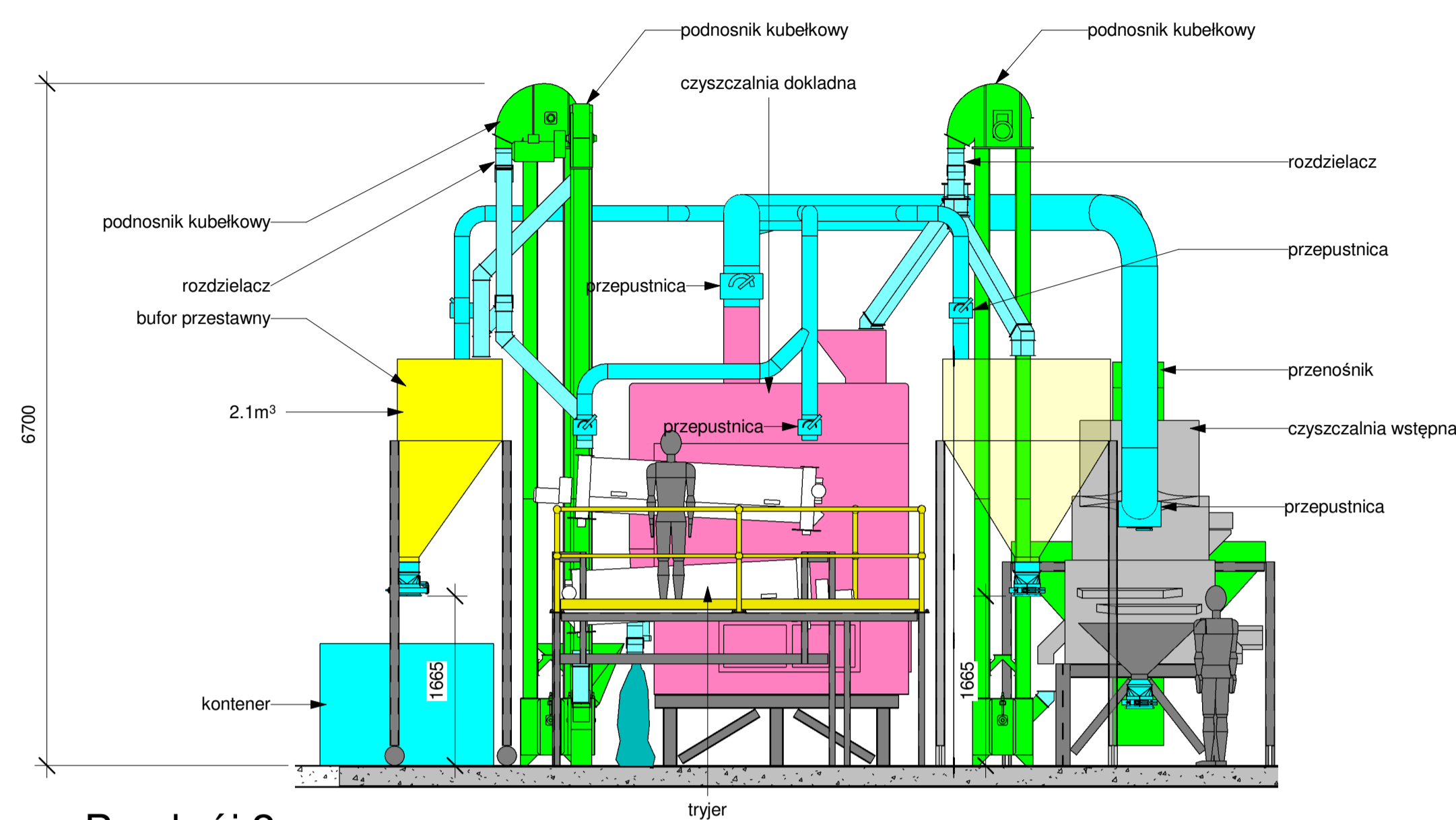
2 Przekrój 2 1 : 50
